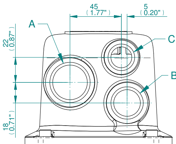
CONDUIT ENTRIES
