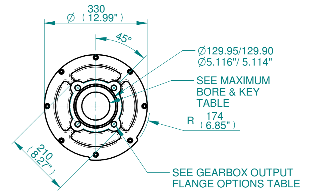
VIEW A-A
