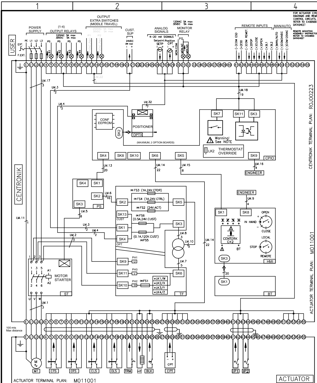
ACTUATOR TERMINAL PLAN: MO11001
