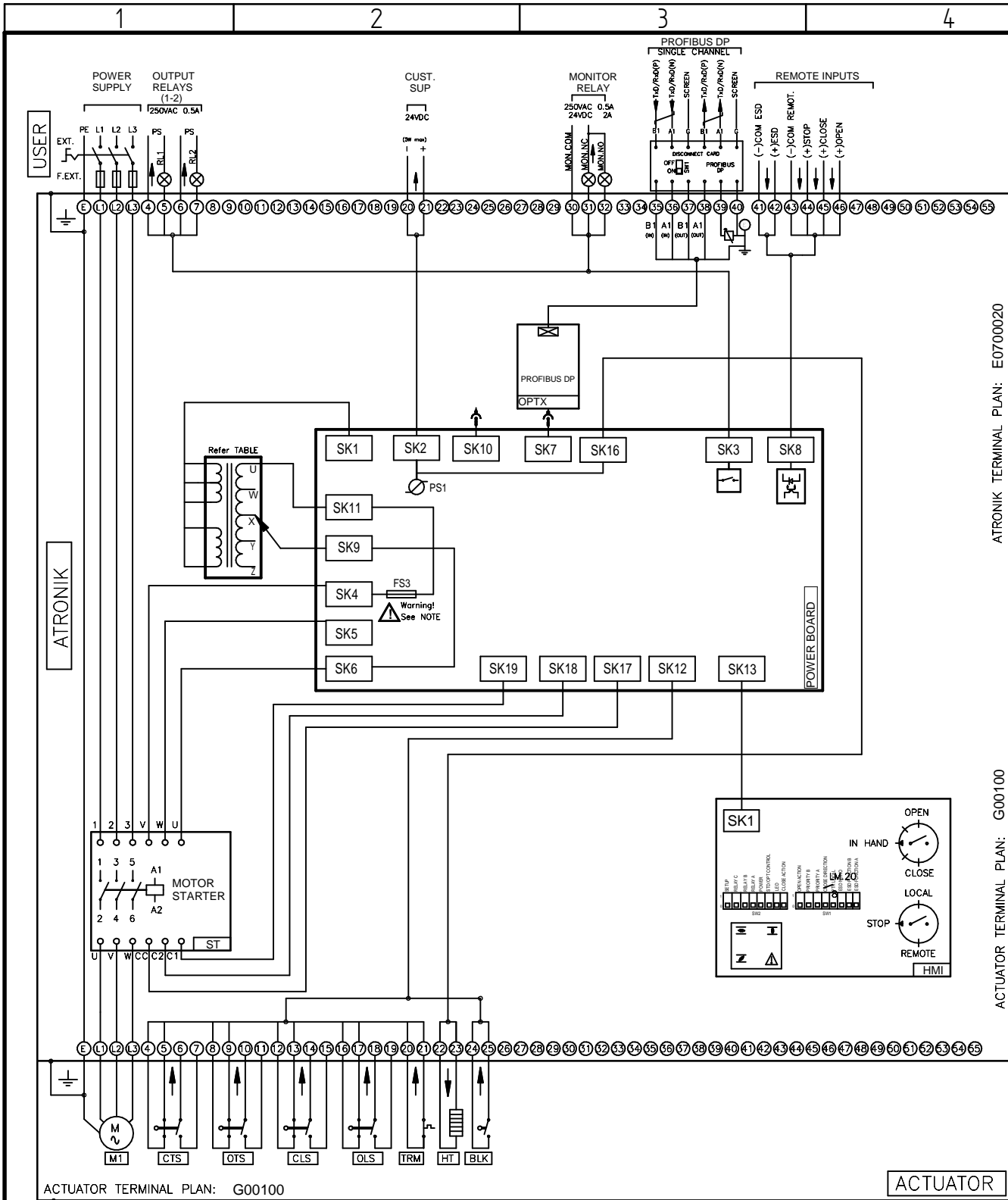
ACTUATOR TERMINAL PLAN: G00100
