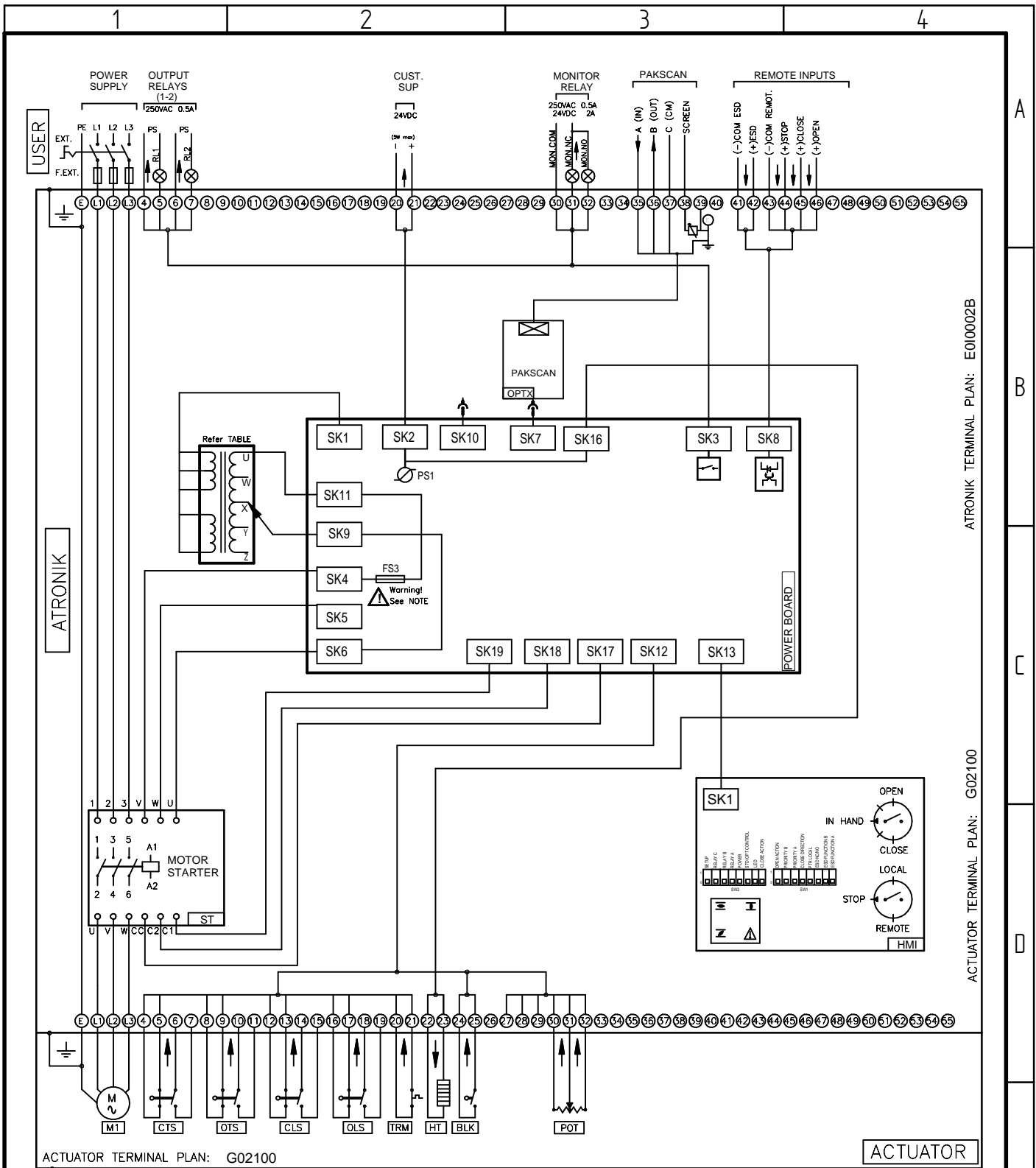
ACTUATOR TERMINAL PLAN: G02100
