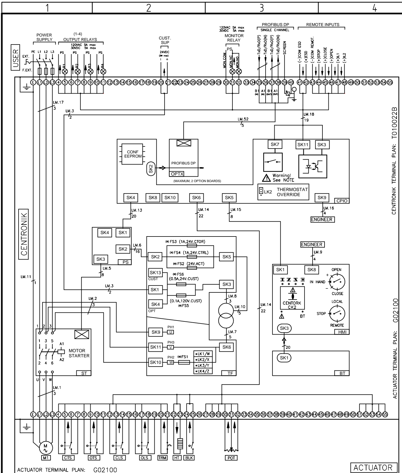
ACTUATOR TERMINAL PLAN: G02100
