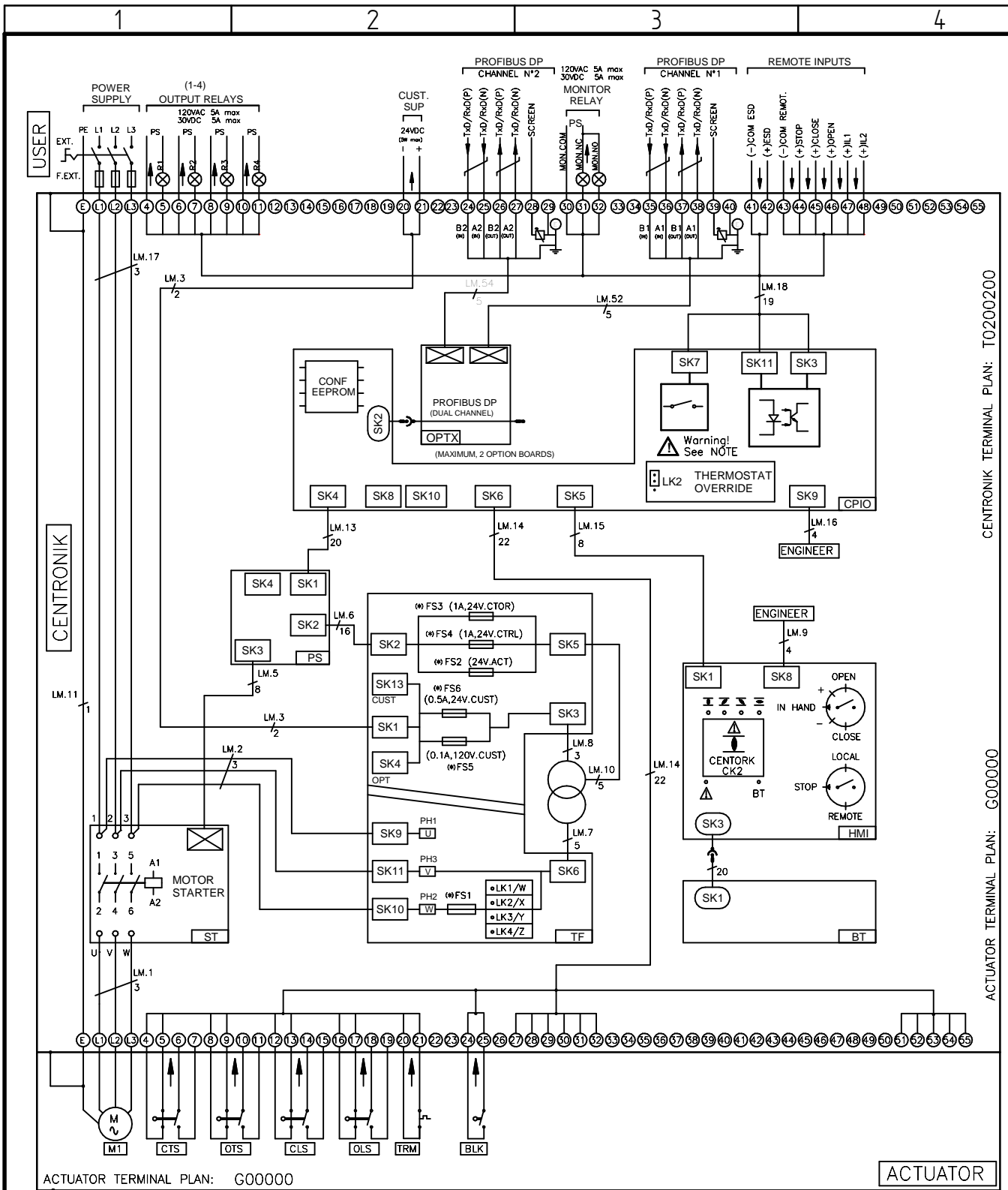
ACTUATOR TERMINAL PLAN: G00000
