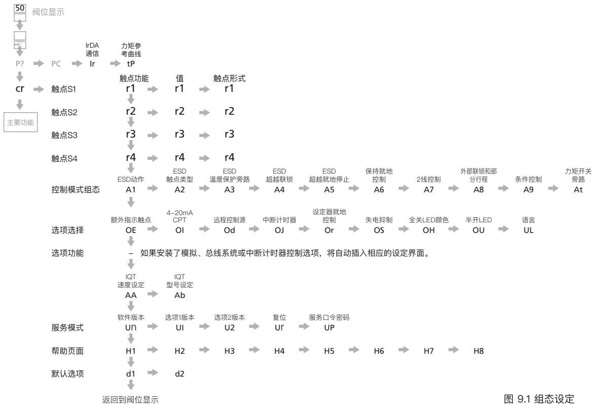
图 9.1 组态设定
