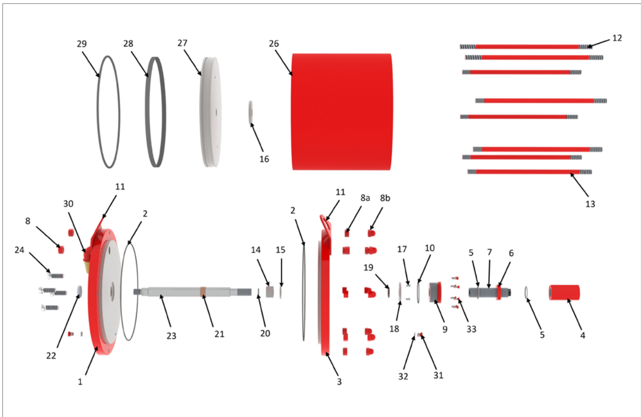
Fig 17.6 Pneumatiske cylindere
