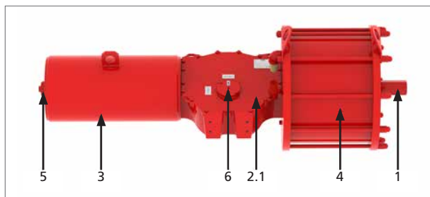
Fig 12.1 GPIS (støbt krop) hovedkomponenter
